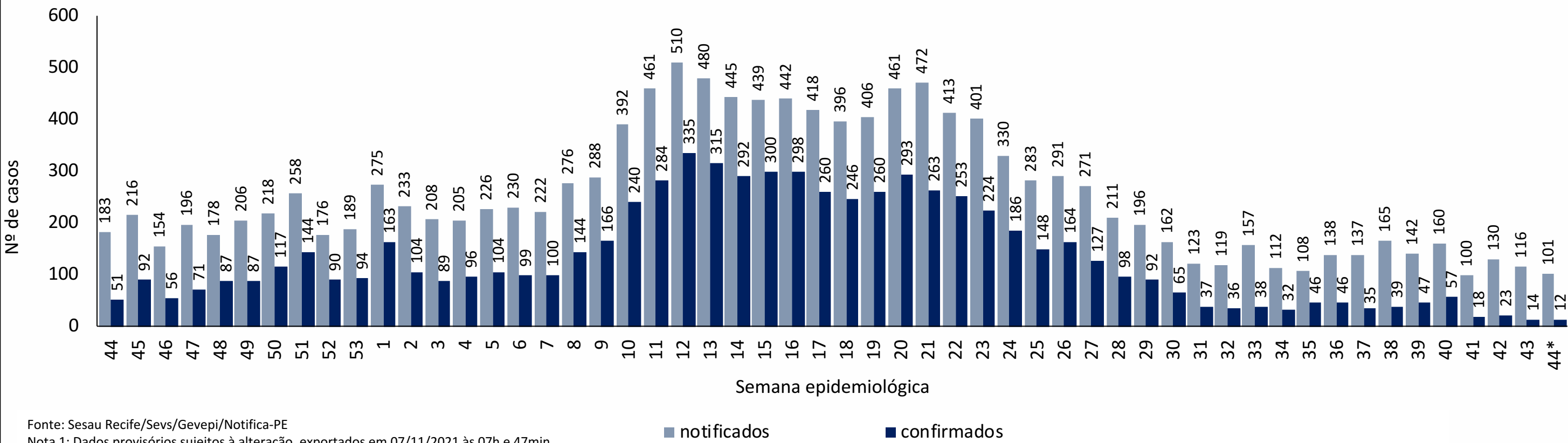
Figura 12. Distribuição dos casos de SRAG, notificados e confirmados para Covid-19, por semana epidemiológica de notificação. Recife, 2020-2021 (até a SE 44*/2021)
