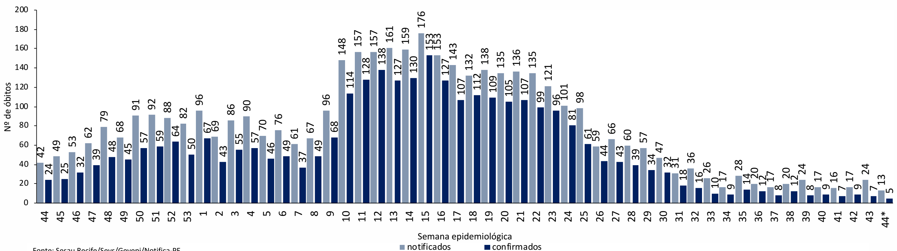
Figura 17. Distribuição dos óbitos de SRAG, notificados e confirmados para Covid-19, segundo semana epidemiológica da ocorrência do óbito. Recife, 2020-2021 (até a SE 44*/2021)
