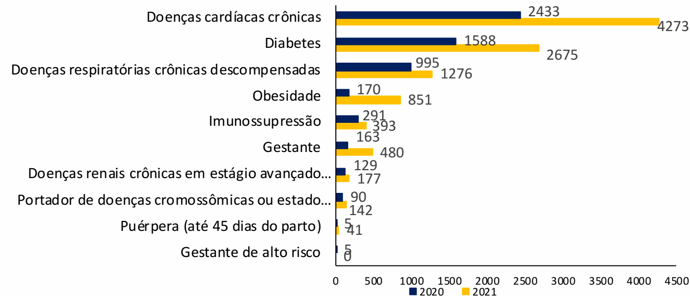
Figura 6. Número de casos leves confirmados para Covid-19, segundo morbidades ou condições prévias. Recife, 2020-2021
