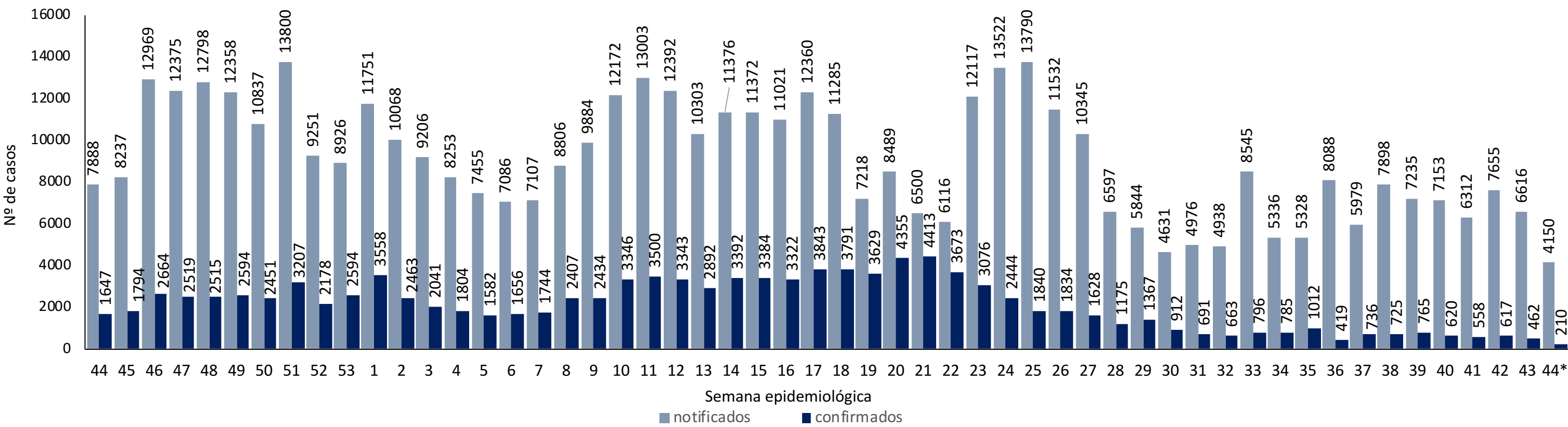
Figura 5. Distribuição de casos leves notificados, confirmados de Covid-19, por semana epidemiológica de notificação. Recife, 2020-2021 (até a SE 44*/2021)
